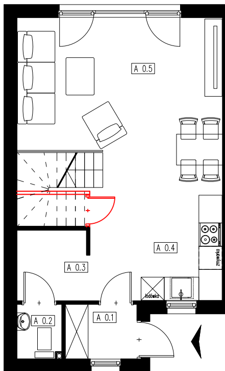
RZUT PARTERU
