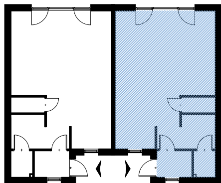
RZUT BUDYNKU
