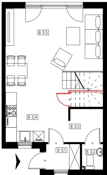
RZUT PARTERU
