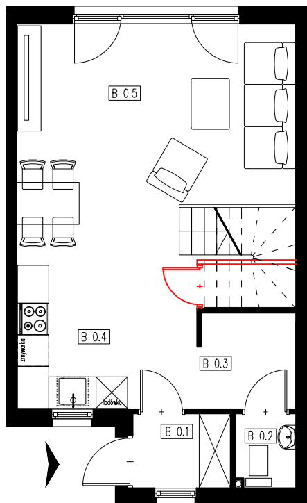
RZUT PARTERU
