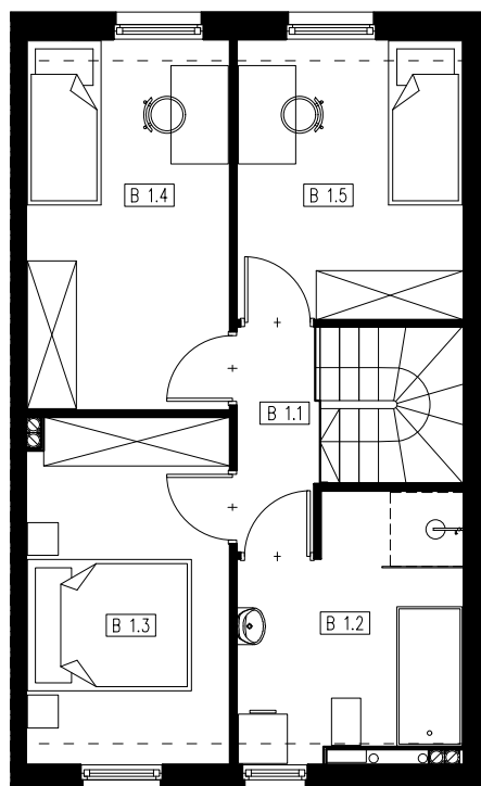
RZUT PIĘTRA
